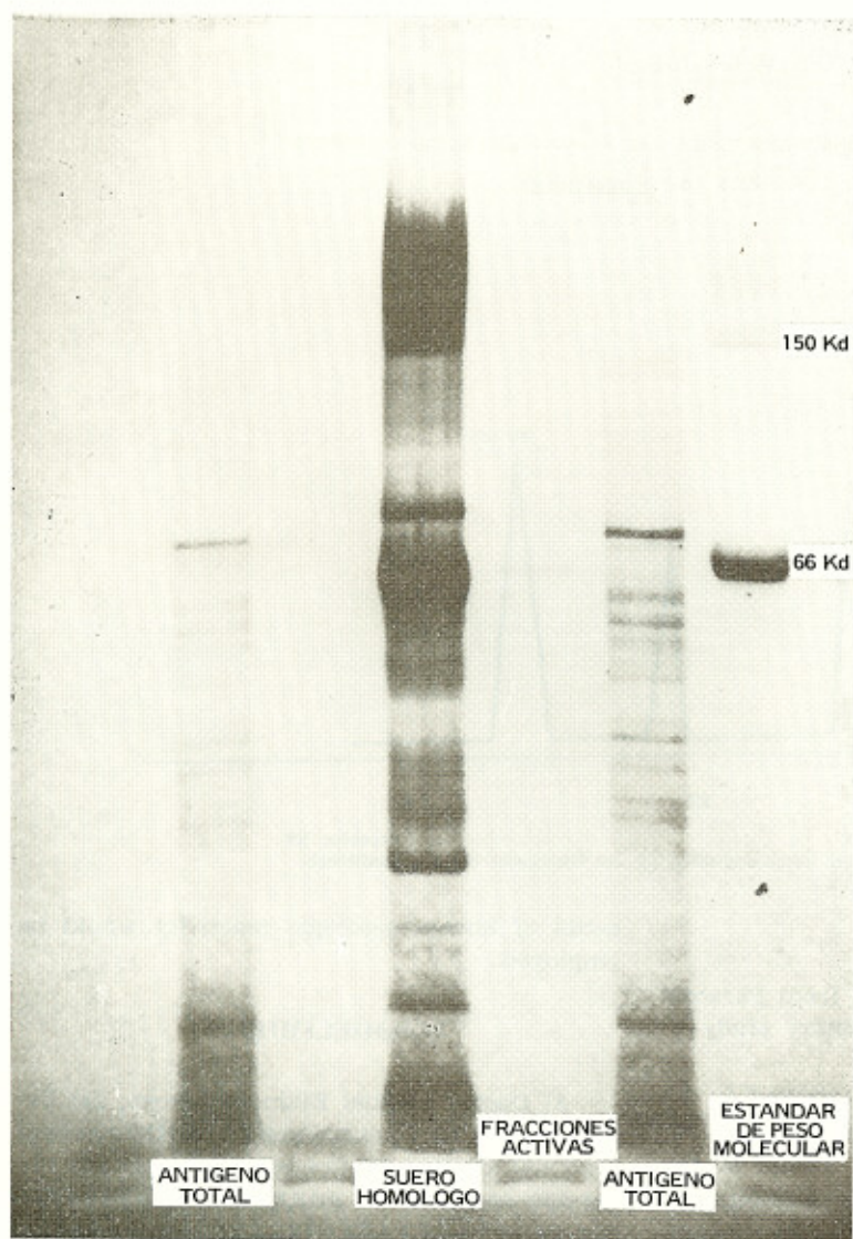
Fig. 1 — Gel de poliacrilamida coloreado con plata. Se observa en la fracción purificada una banda de precipitado de peso molecular aproximado de 66 kd
