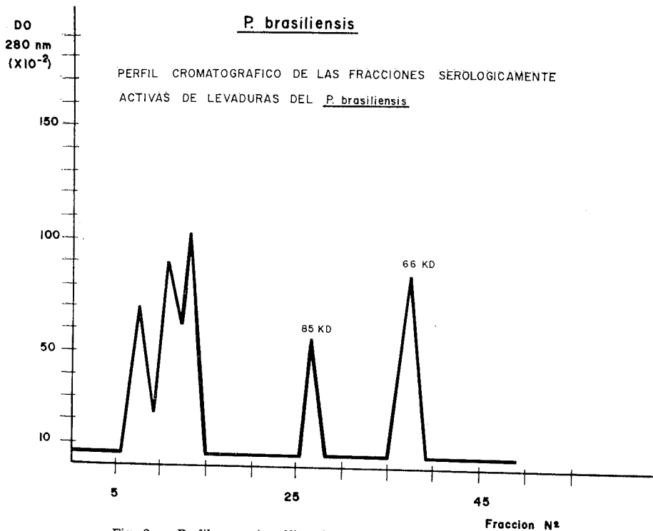
Fig. 2 — Perfil cromatográfico de las fracciones del P. brasiliensis
